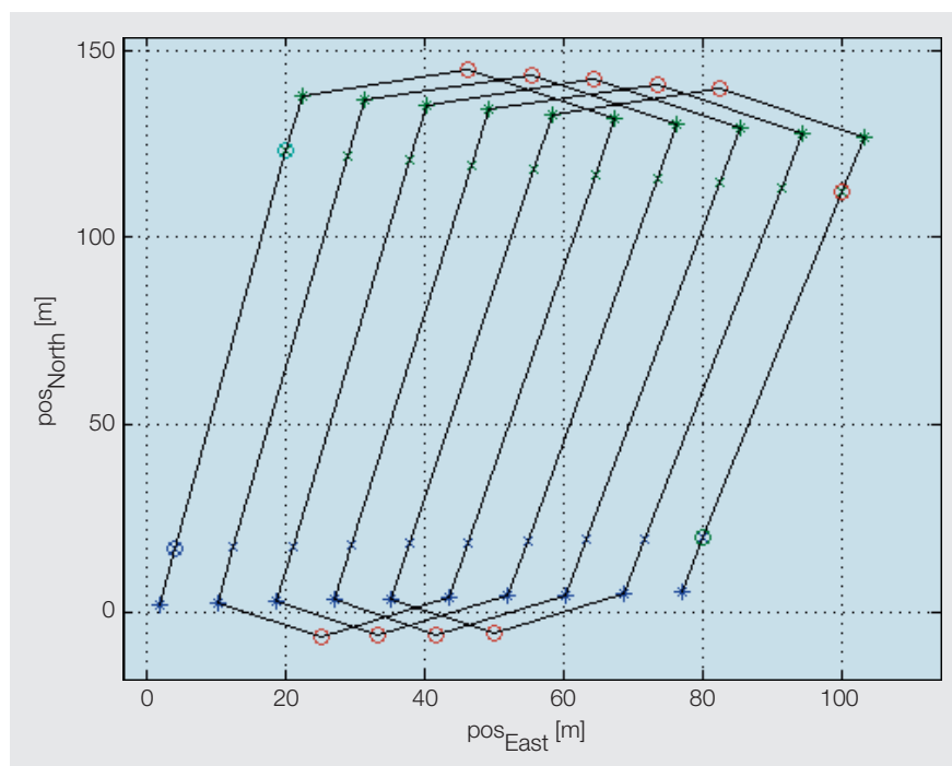
Bild 3 Ein Beispiel für die Flugplanung mit mehreren Fluglinien, die jeweils mit GPS-Positionskoordinaten vorgegeben sind.
