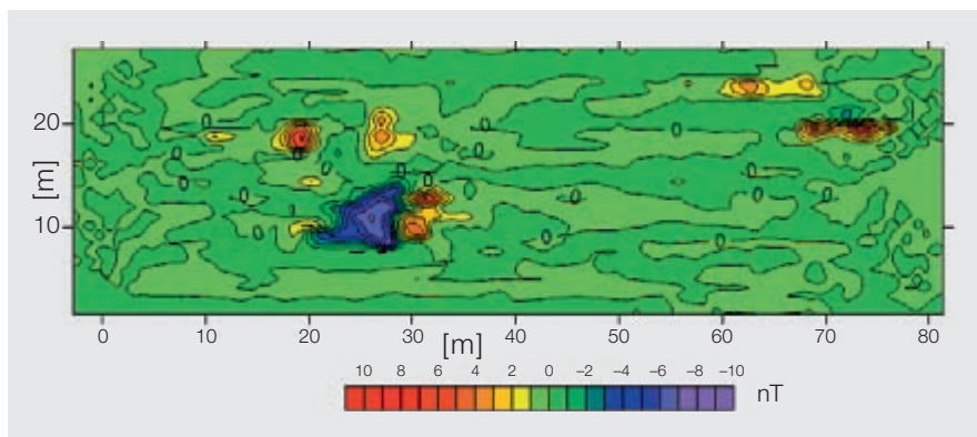
Bild 6 Resultierende magnetische Feldstärke, die bei UAV-basierten Messungen erzielt werden konnte. Die detektierten Objekte sind deutlich zu erkennen.
